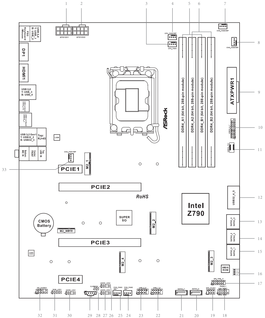
上面図
